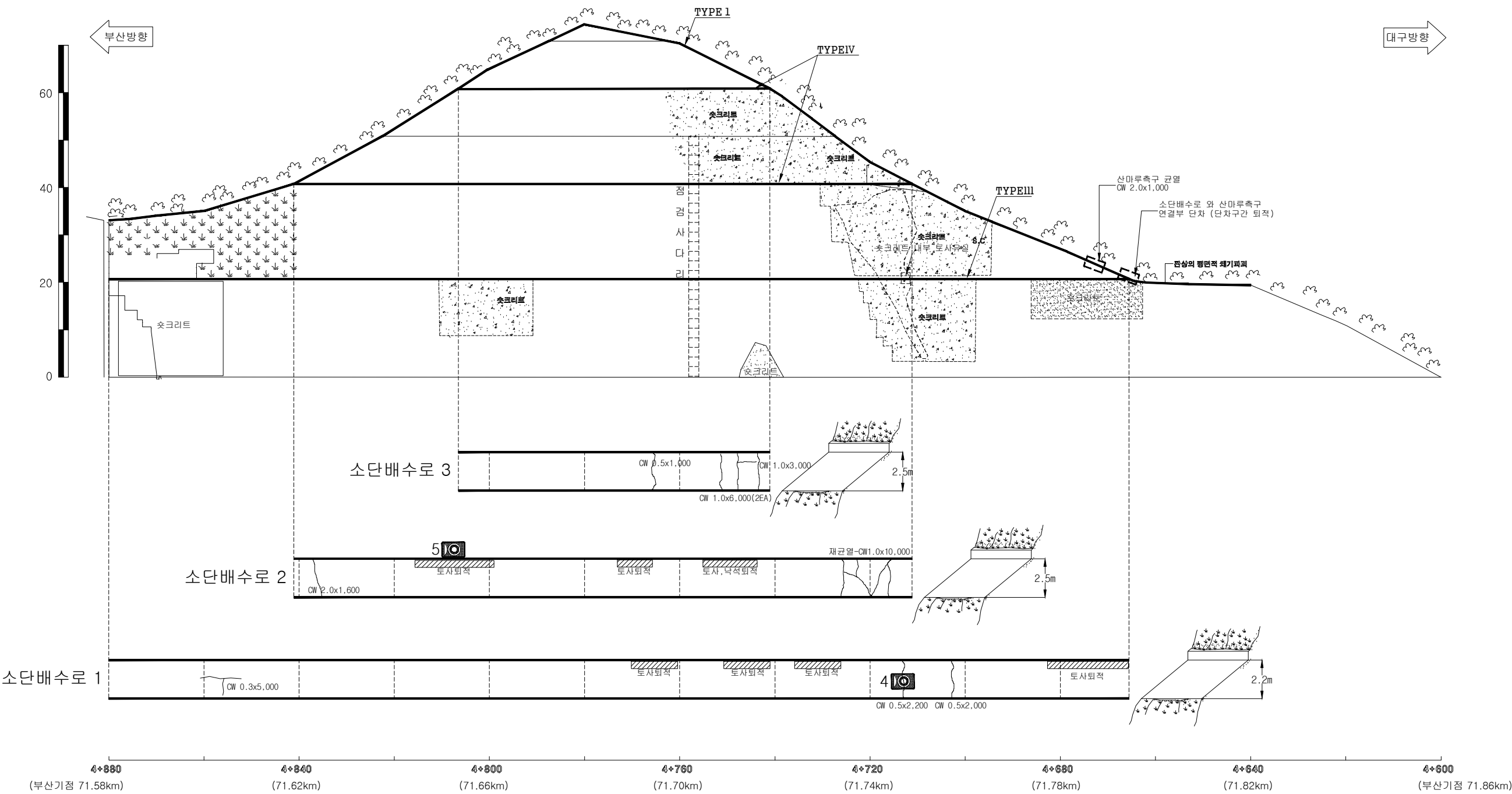
부산절토 16 / 부산기점 71.58~71.86km (4공구 STA.4+600~4+880)
